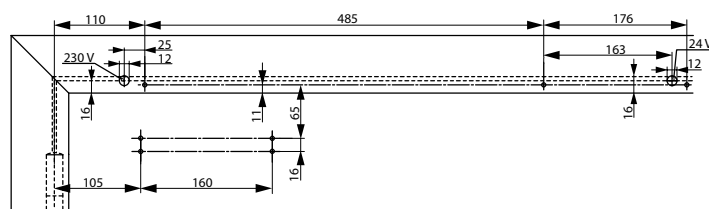
Instalace s montážním plechem na straně proti pantům
