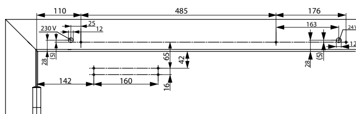
Instalace s montážním plechem na straně pantů
